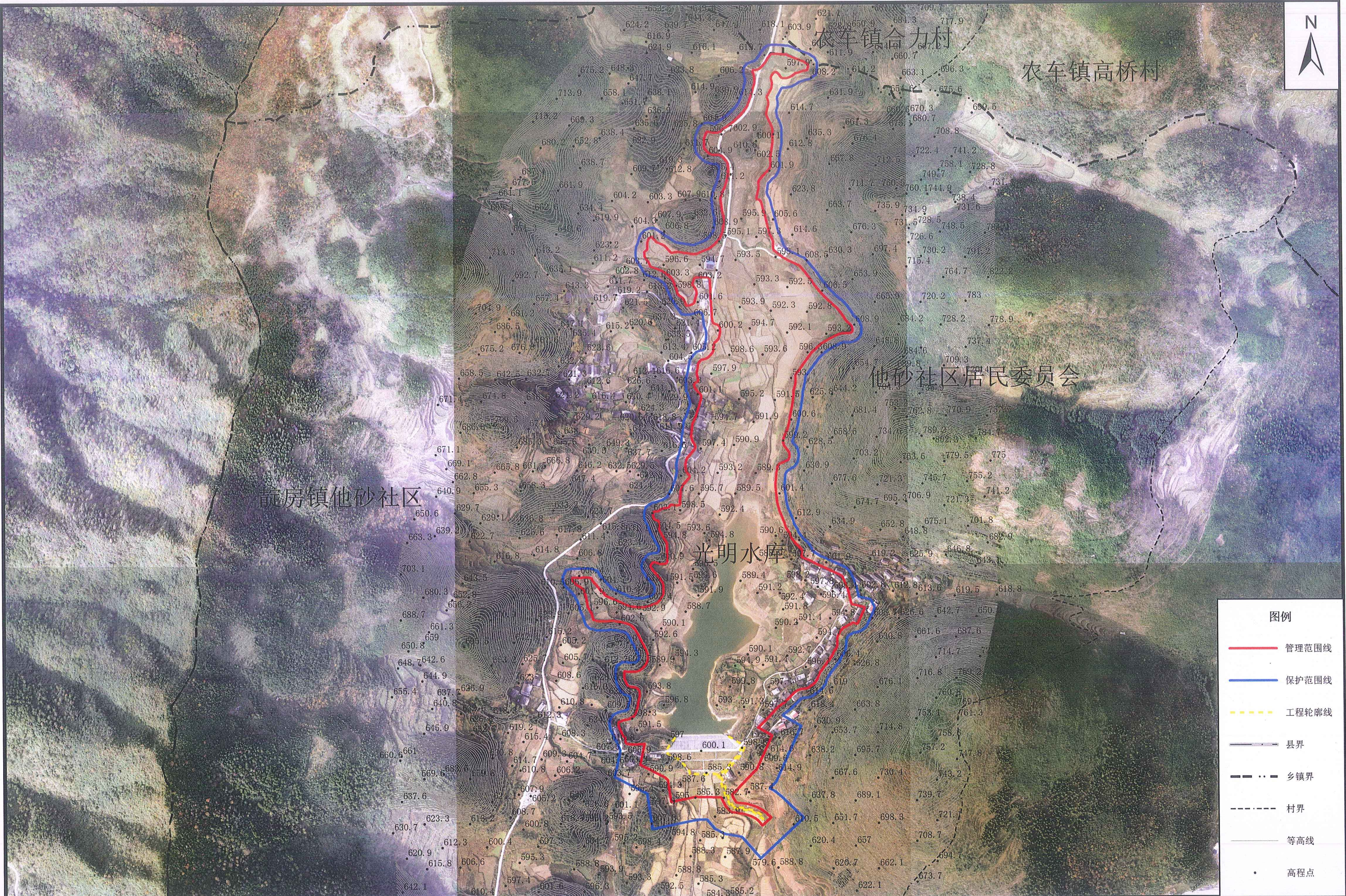
光明水库管理与保护范围划界成果示意图
