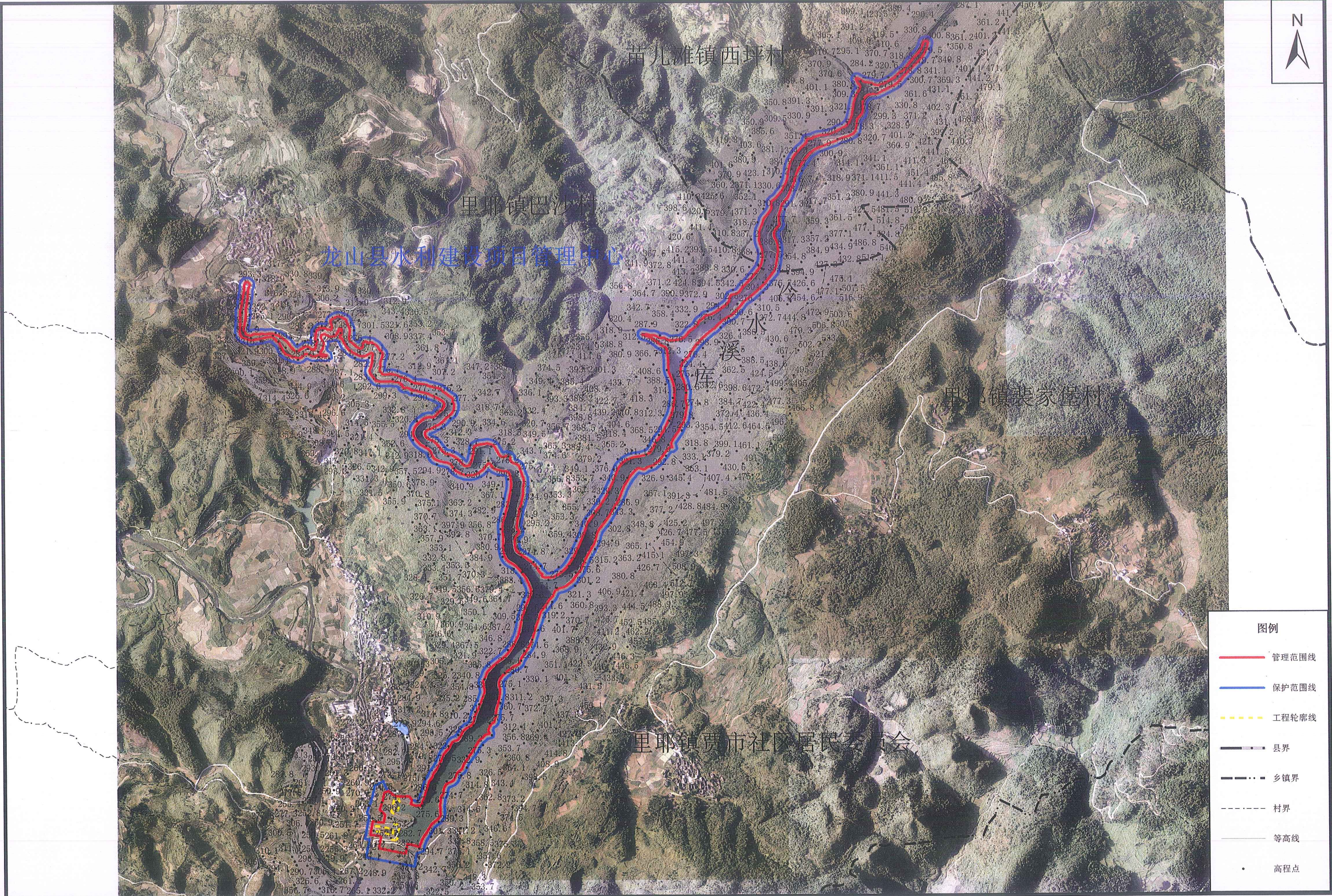
冷水溪水库管理与保护范围划界成果示意图
