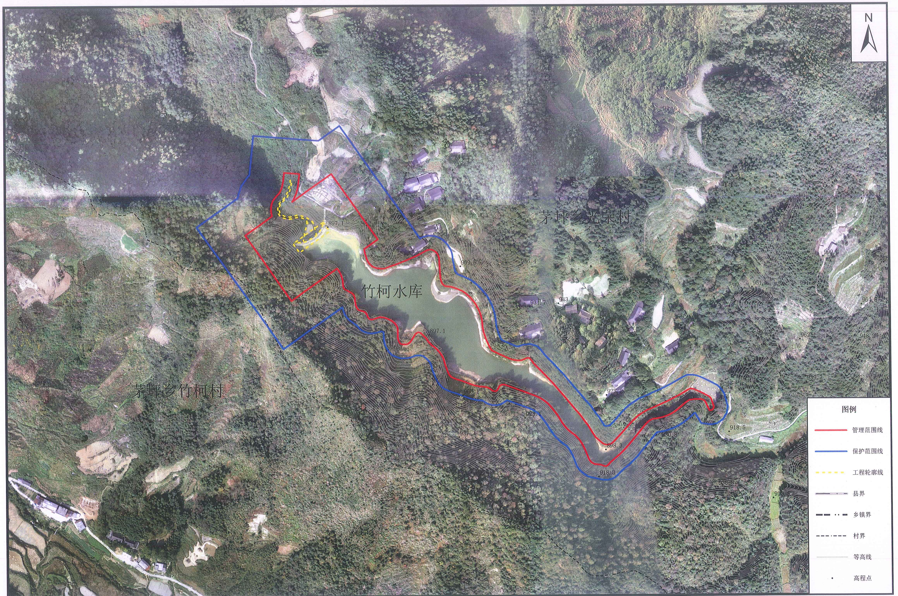
竹柯水库管理与保护范围划界成果示意图
