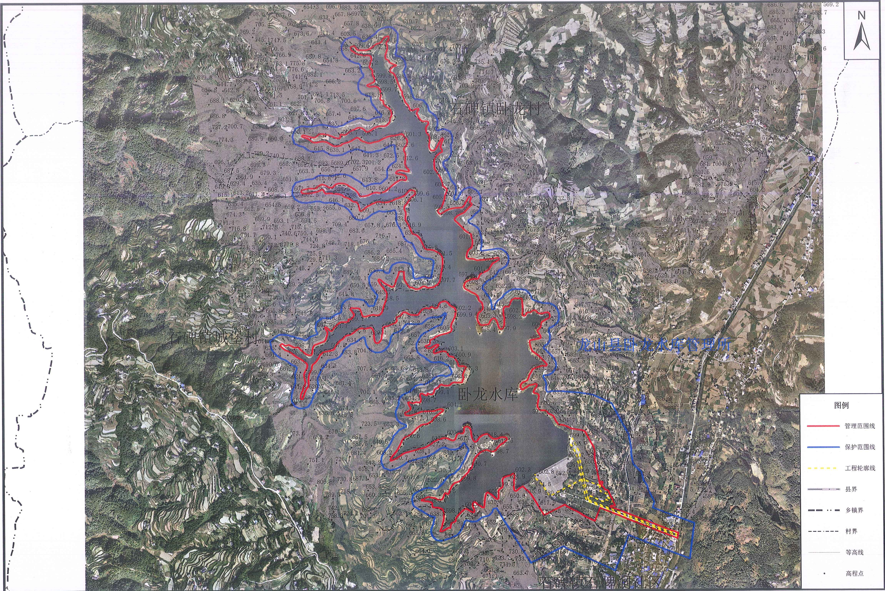
卧龙水库管理与保护范围划界成果示意图
