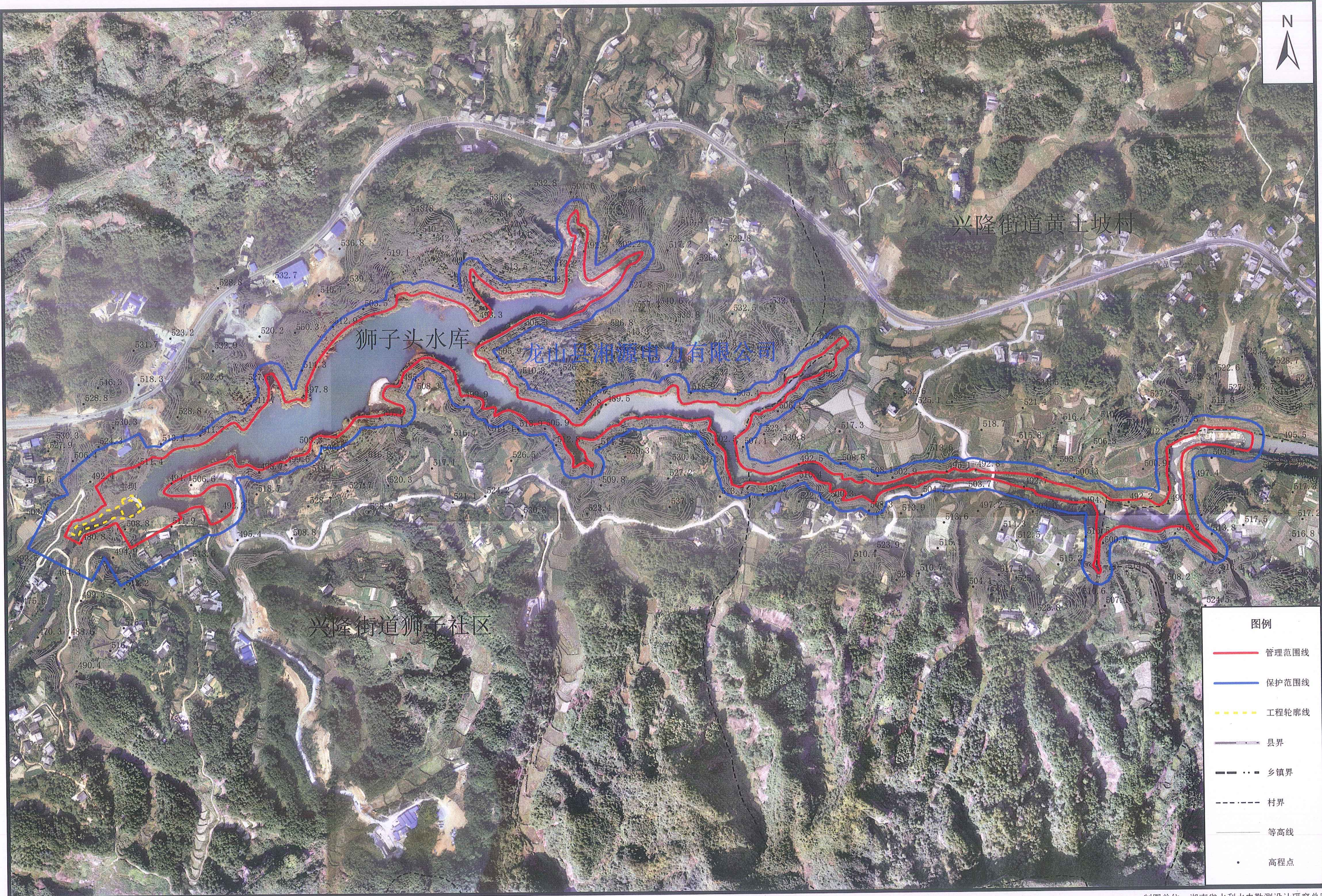
狮子头水库管理与保护范围划界成果示意图
